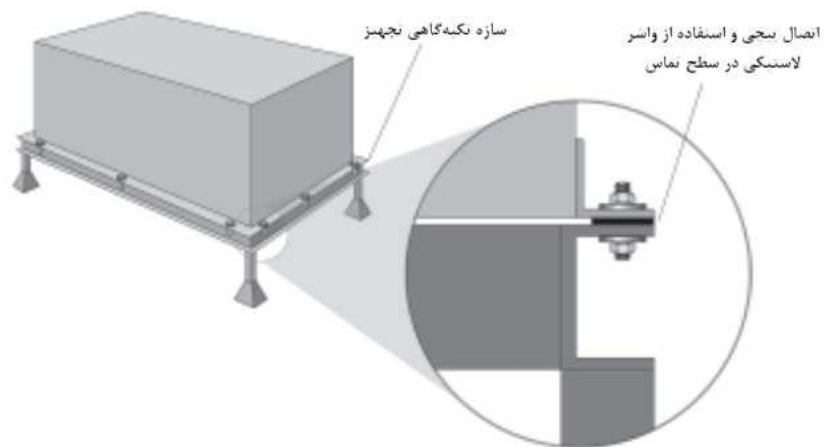
شکل ۲۱-۷-۱- نمونه‌ی اتصال تجهیز به سازه نکیه‌گاهی
