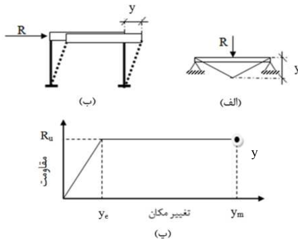
شکل ۳-۵-۲۱- سازه یک‌درجه آزادی ارتجاعی - خمیری
