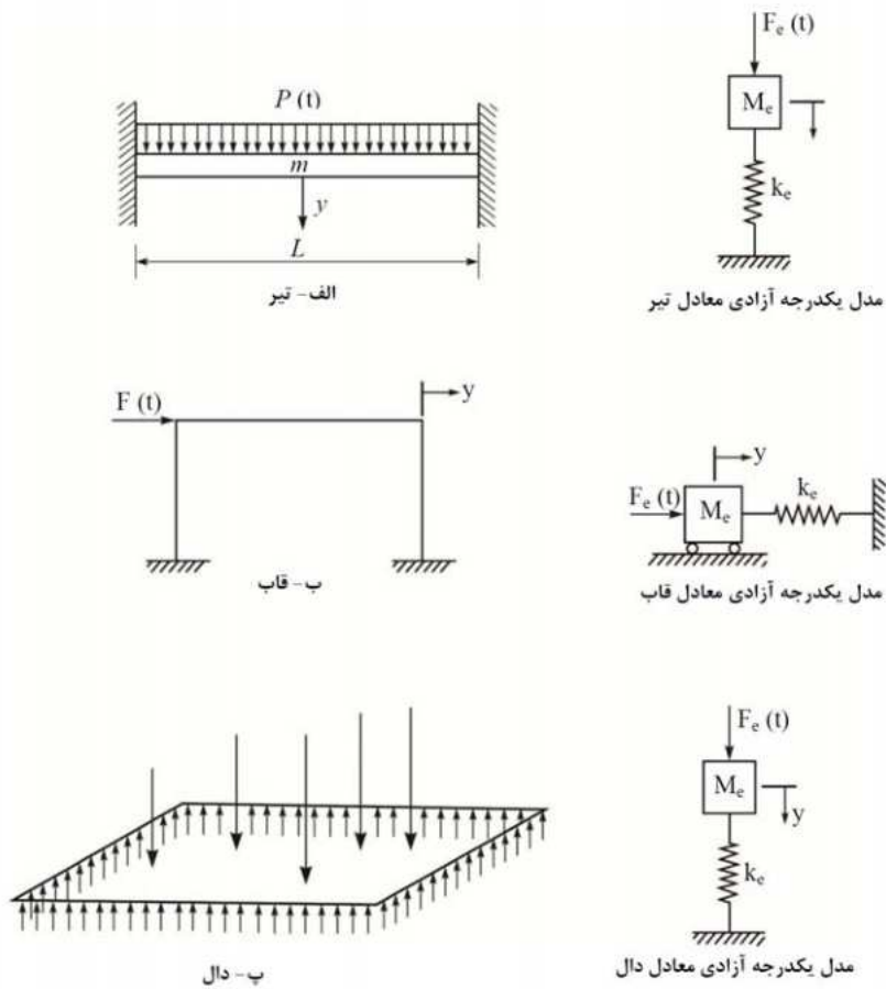
شکل ۲۱-۵-۱- معادل سازی سازه‌ها با مدل یک‌درجه آزادی
