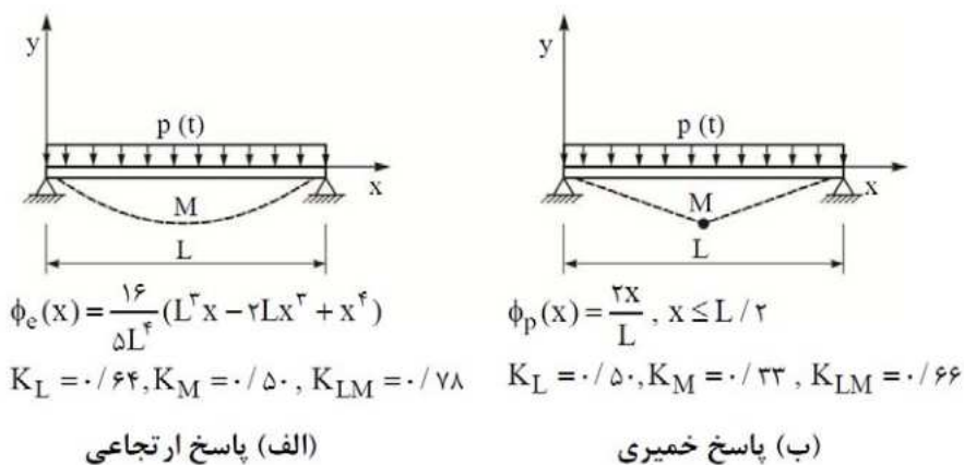
شکل ۴-۵-۲۱- تابع شکل و ضرایب انتقال برای تیر دو سر ساده
