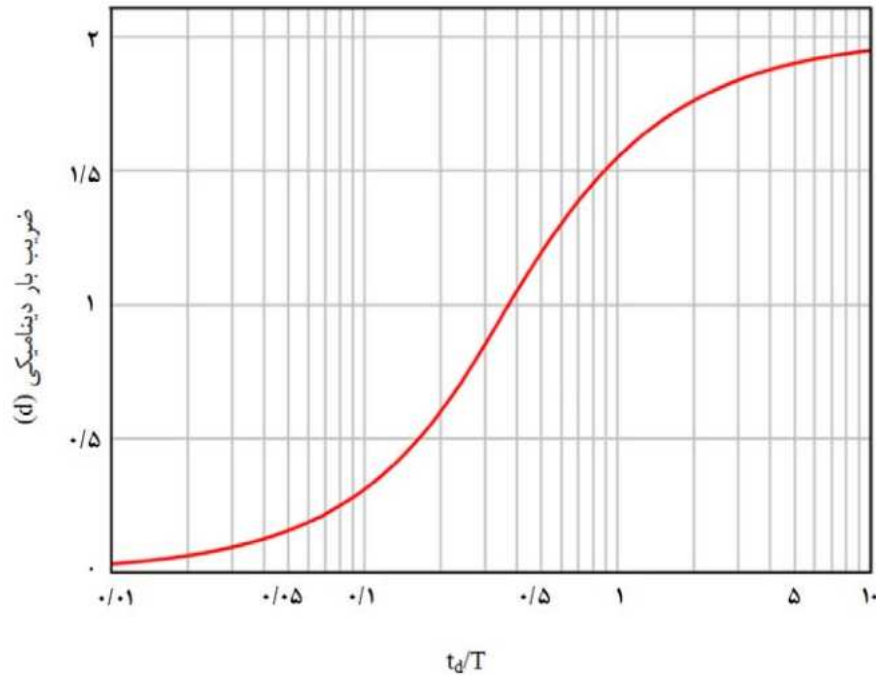
شکل ۶-۵-۲۱- ضریب بار دینامیکی برای انفجار با فاصله
