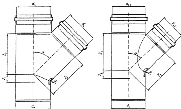
سه راه ۴۵ درجه با دو سرکاسه
