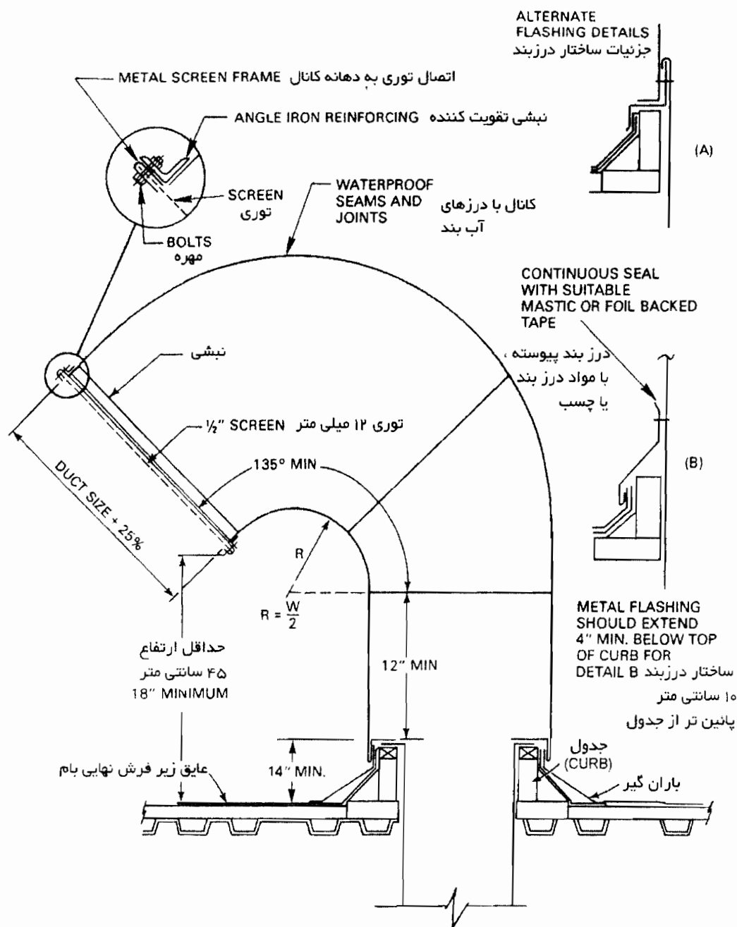
شکل شماره (۵-۷-۴-۲) "ب" کانال دهانه ورود یا تخلیه هوا (گردن غازی)
