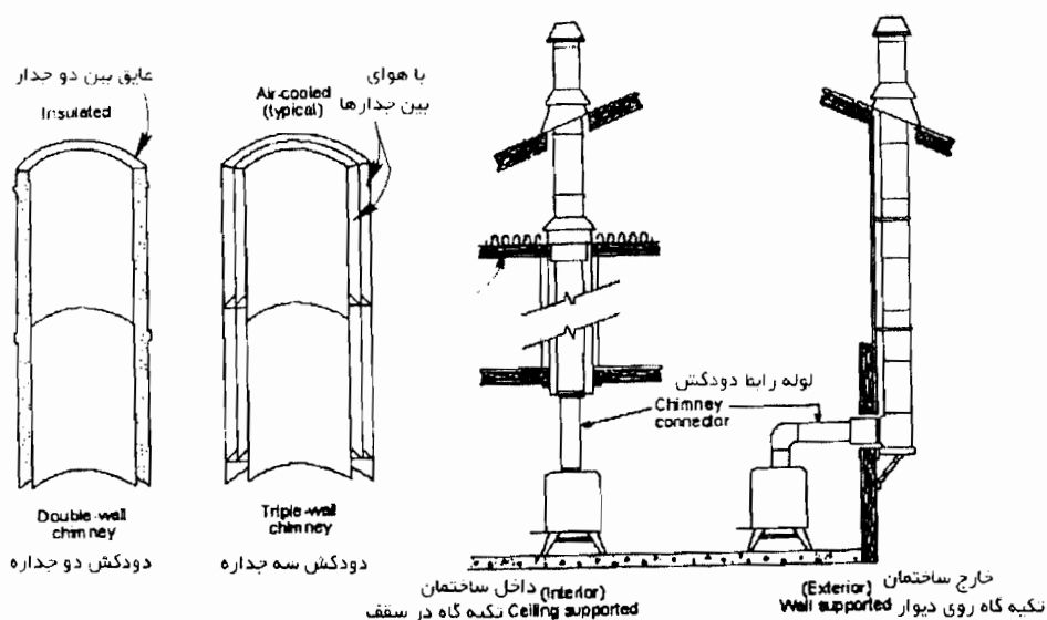
شکل شماره (۴-۱۰-۵) "ب" (۳) نمونه هایی از دودکش پیش ساخته (خانگی)
