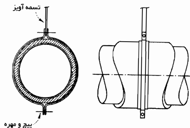
شکل شماره (۴-۸-۴-۲) "ب" (۳) آویز و بست کانال گرد افقی، بست خارج از عایق
