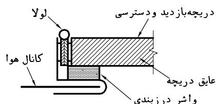
چهارچوب و لولای تیپ ۲
