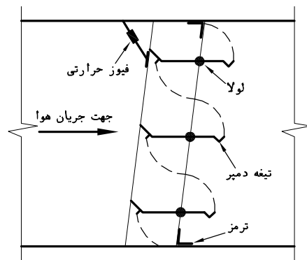
شکل ۳- دمپر آتش چند تیرغه‌ای
