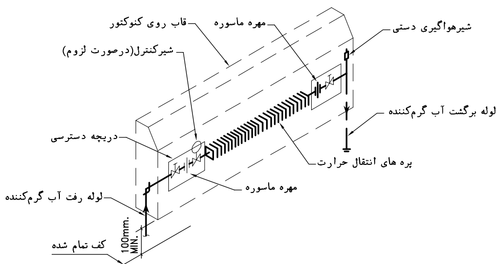
دیاگرام لوله کشی کنوکتور در حالت تغذیه از پائین (UP-FEED CONNECTION)
