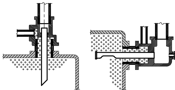
جداکننده هوا برای نصب روی دیگ
