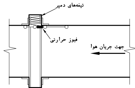
شکل ۳- دمپر آتش چند تیرغه‌ای
