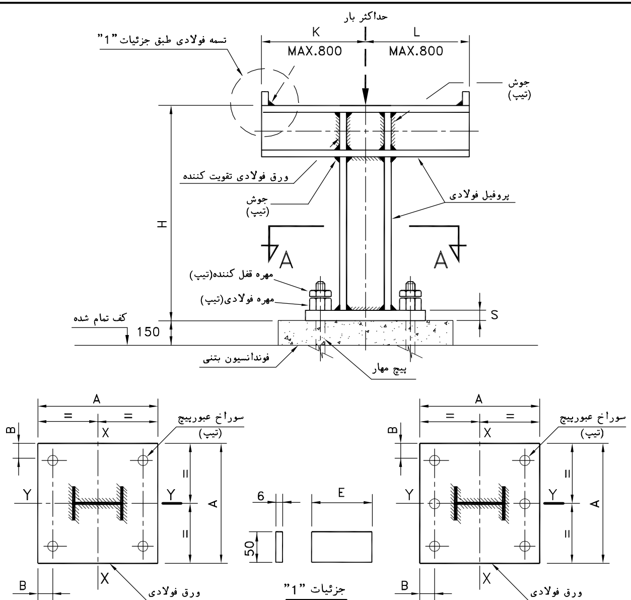
مقطع A-A برای تکیه گاههای شماره ۳ و ۲
