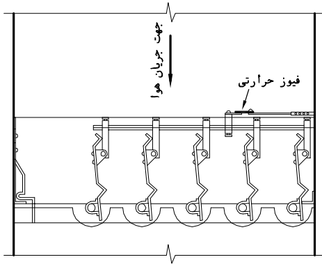
شکل ۴- دمپر آتش چند تیرغه‌ای
