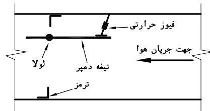
شکل ۱- دمپر آتش لولائی یک تیرغه‌ای
