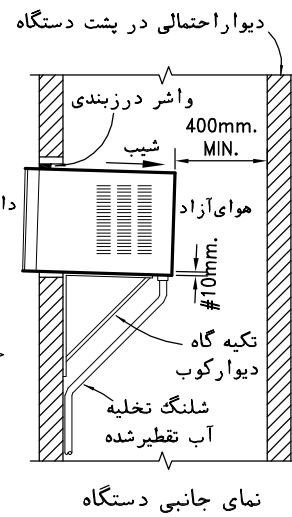
بازشو نصب دستگاه، روی دیوار با ضخامت کم
