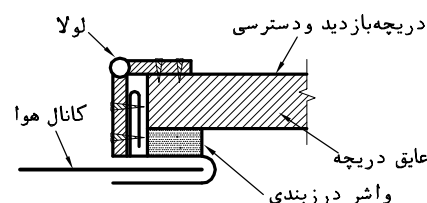
چهارچوب و لولای تیپ ۳
